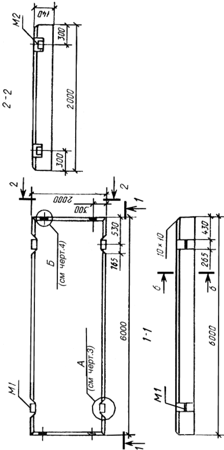
Плита ПАГ-18 и ПАГ-20
